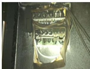
Smeltet elmåler.
