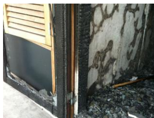
Udbrændt vindue.
